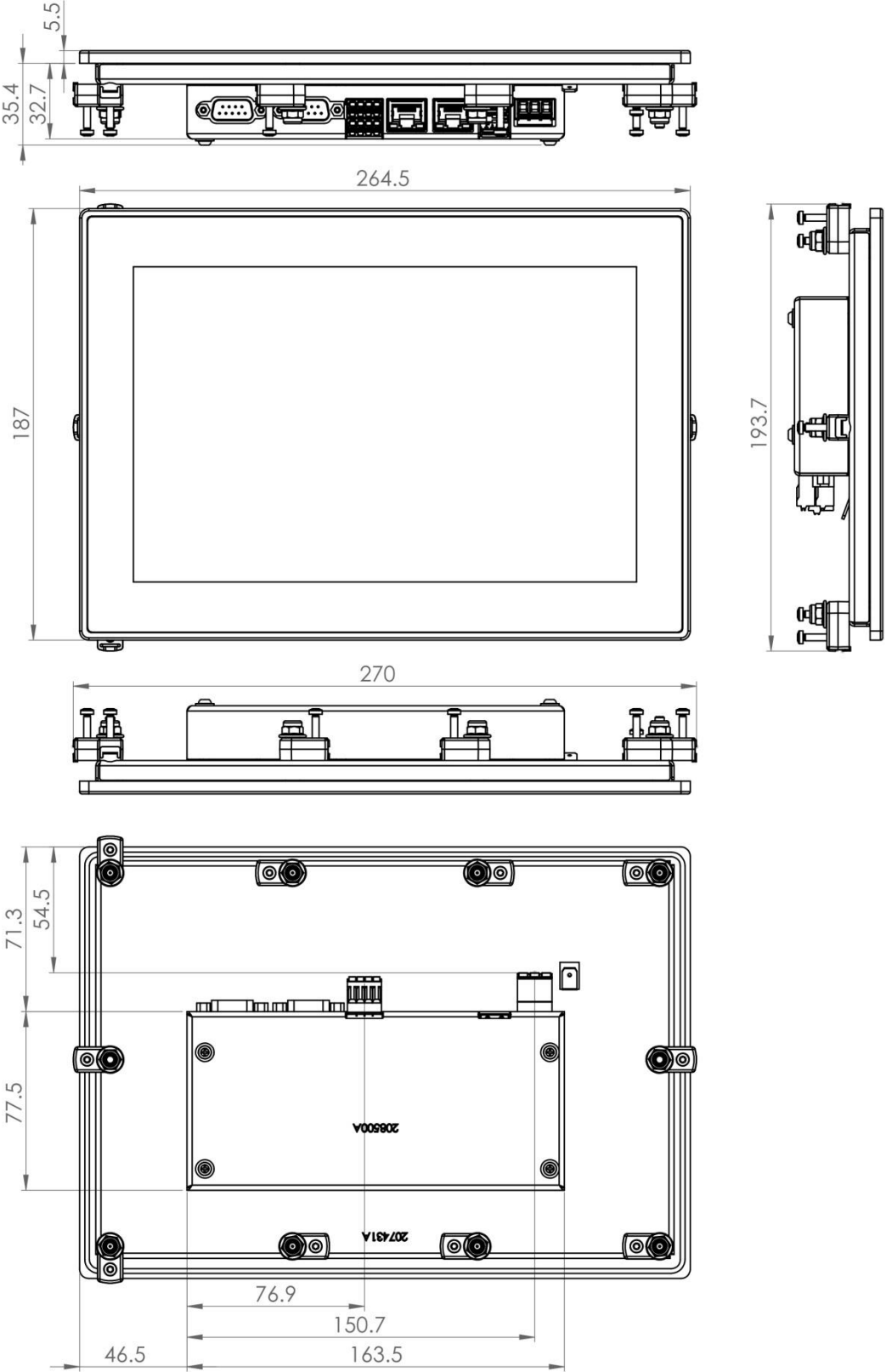
Bild 7: Maßzeichnungen
