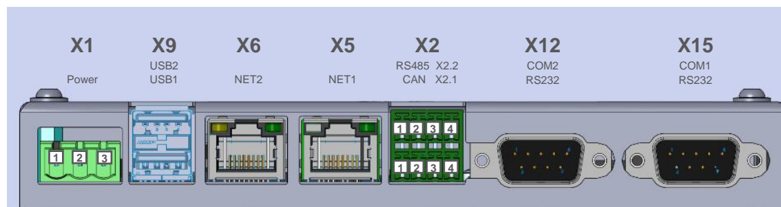
Bild 2: Schnittstellen unten bei Control Panels CP-101g 3x-xx30
