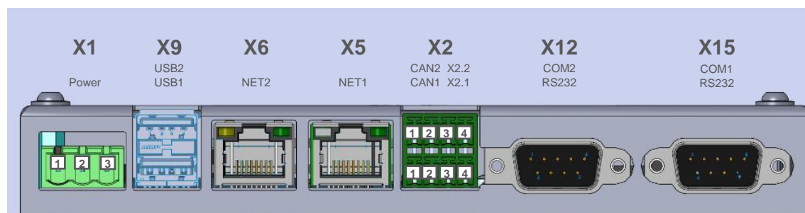
Bild 3: Schnittstellen unten bei Control Panels CP-101g 3x-xx40
