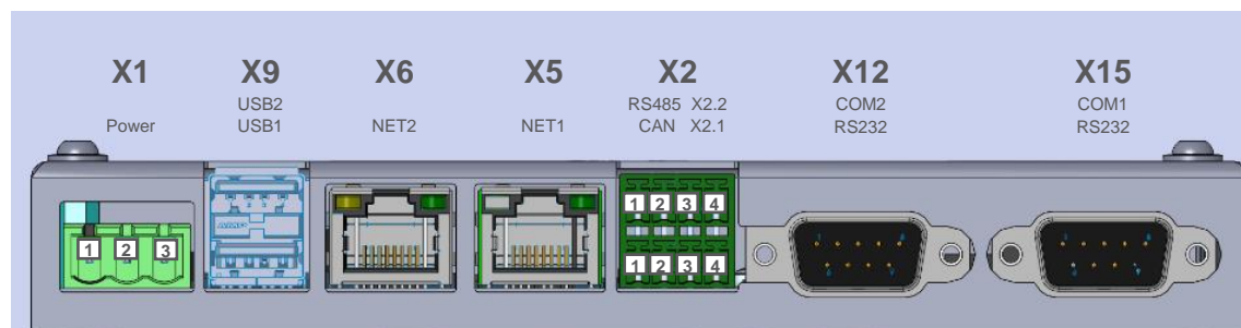
Bild 2: Schnittstellen unten bei Control Panels CP-70g 3x-xx30
