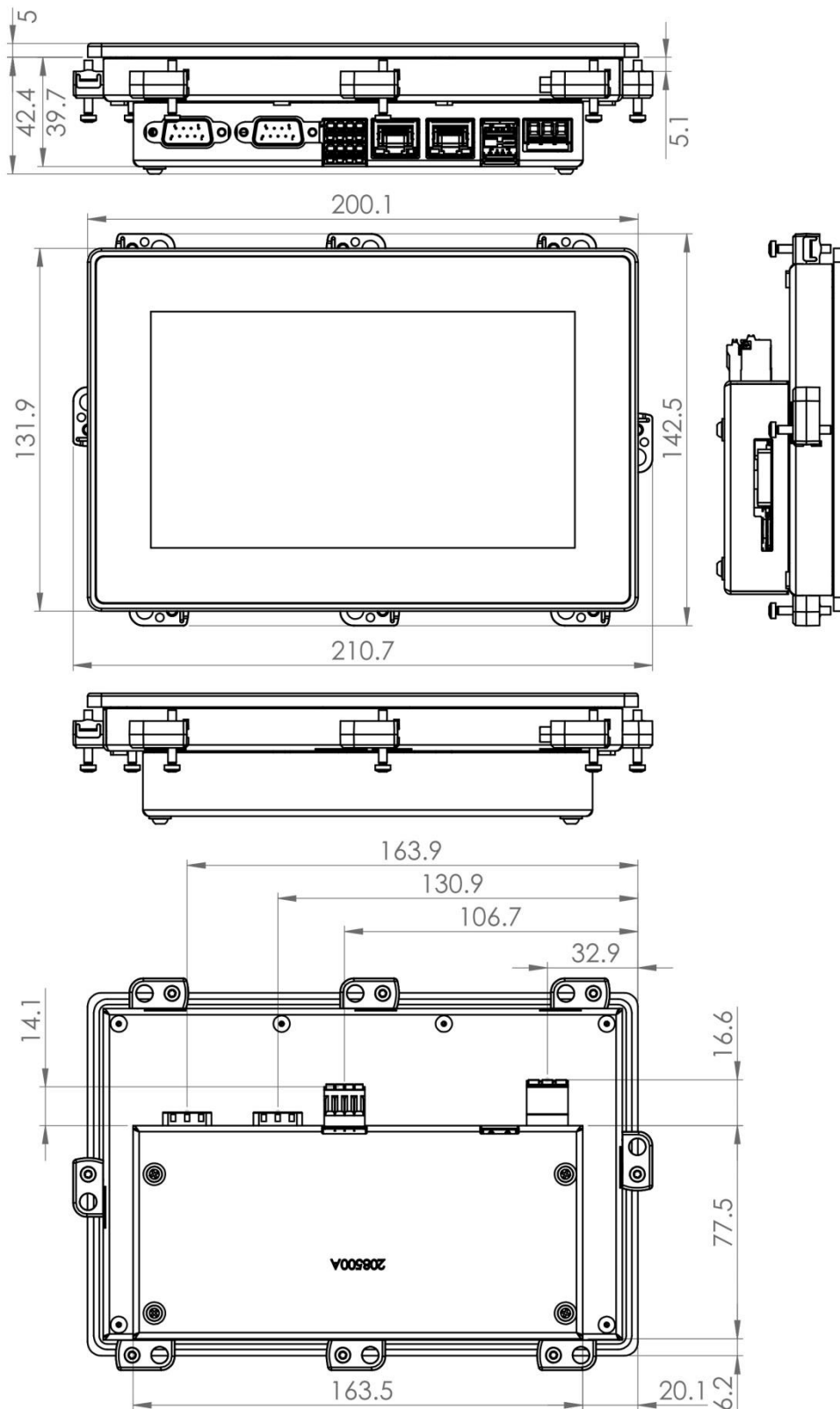
Bild 7: Maßzeichnungen CP-70g 32-12x0 (Versionen mit Aluminiumrahmen)
