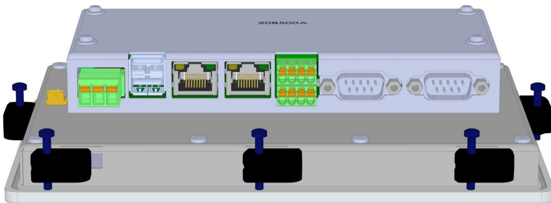
Bild 11: Seitenansicht von unten
