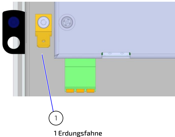
Bild 5: Funktionserdeanschluss bei Control Panels CP-70g 3x-xx40 (2. Möglichkeit)
