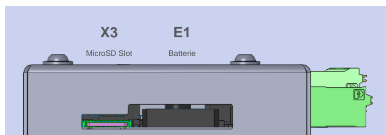
Bild 4: Schnittstellen seitlich
