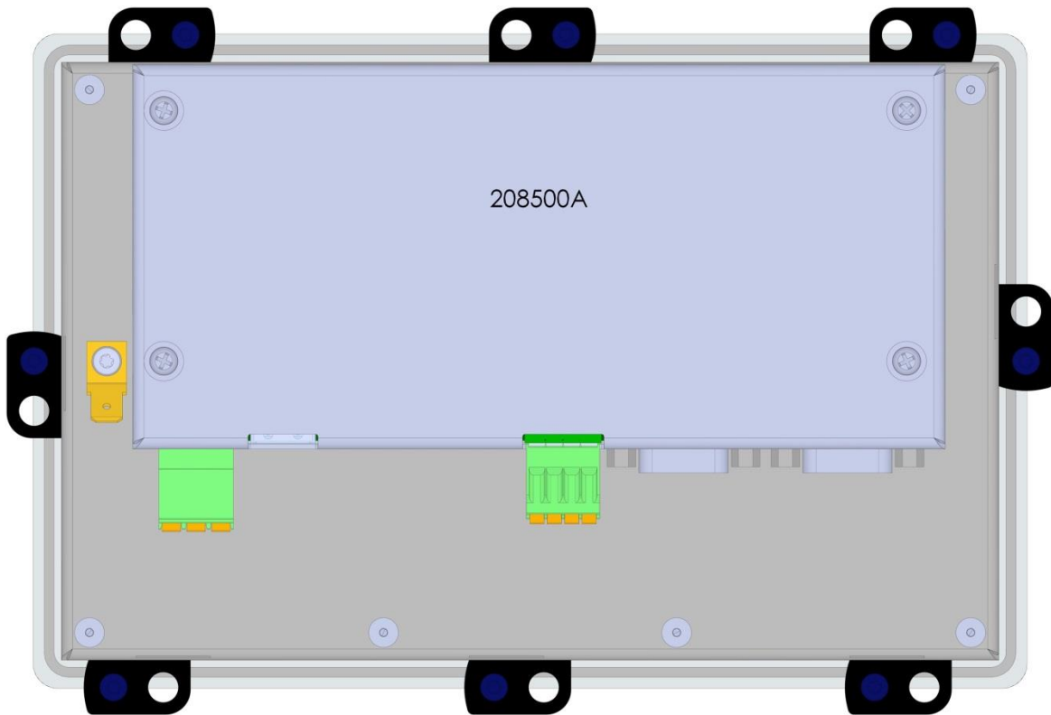
Bild 10: Rückansicht
