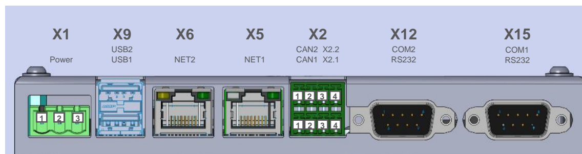
Bild 3: Schnittstellen unten bei Control Panels CP-70g 3x-xx40
