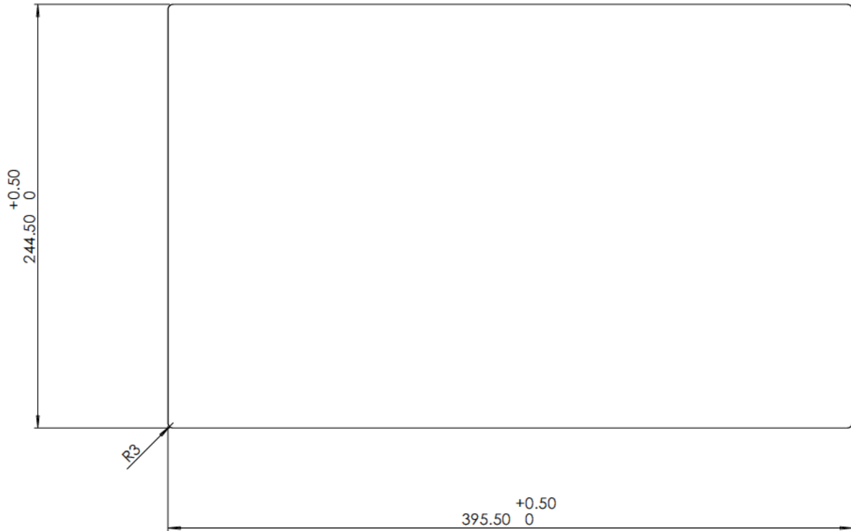
Bild 6: Montage-Ausschnitt
